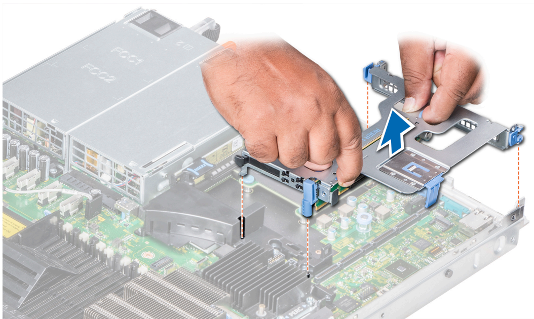
Abbildung 35. Entfernen des Erweiterungskarten-Risers 1A
