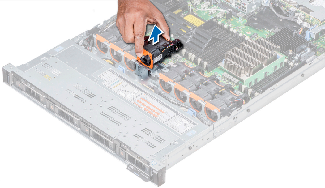
Abbildung 23. Entfernen des Kühl Lüfters
