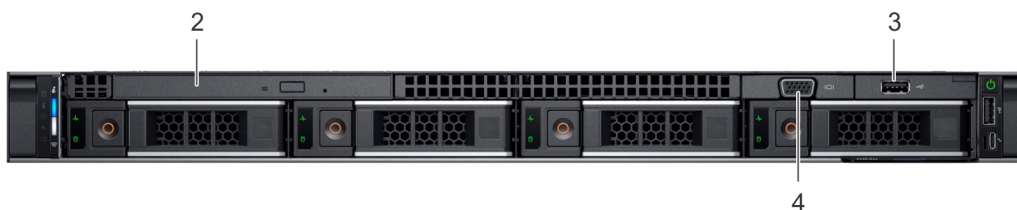
Abbildung 2. Vorderansicht des 4-x-3,5-Zoll-Laufwerks-Systems
