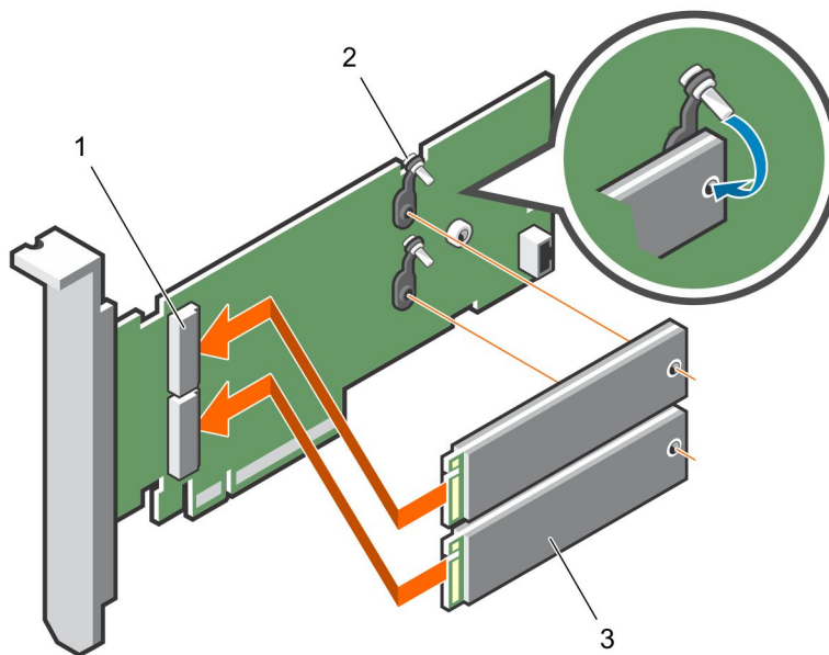
Abbildung 88. Einbau des M.2 SSD-Moduls
