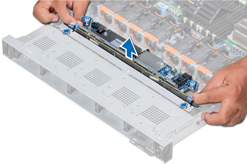
Abbildung 59. Entfernen der Festplatten-Rückwandplatine
