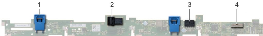
Abbildung 60. 4 x 3,5-Festplatten-Rückwandplatine
