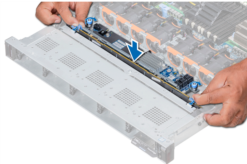
Abbildung 61. Installieren der Festplatten-Rückwandplatine
