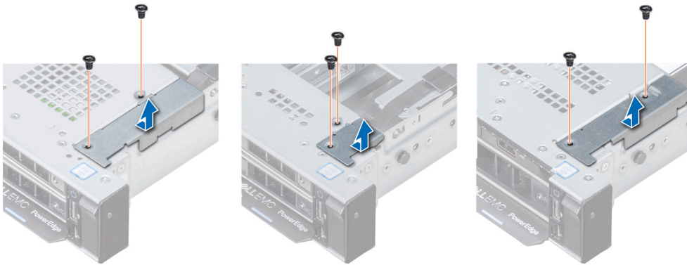
Abbildung 79. Entfernen der Kabelabdeckung
